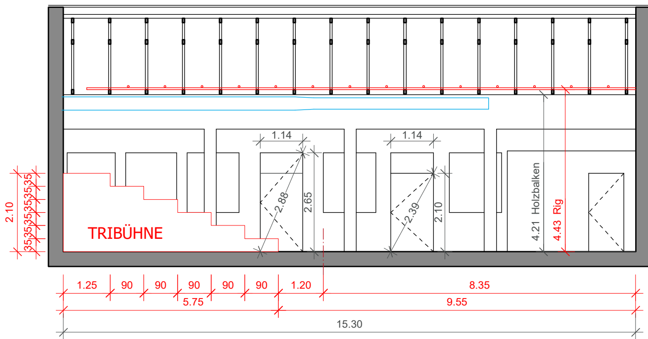
Längsschnitt
